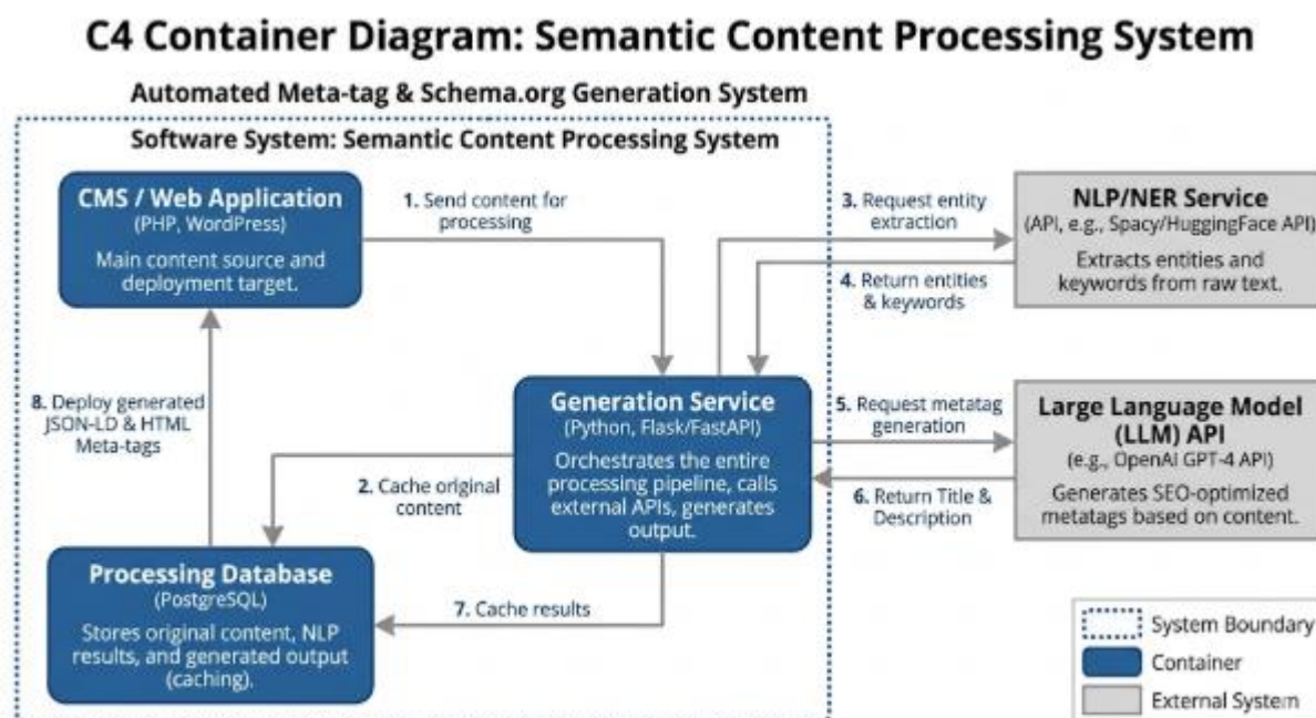
Рис. 1. Архітектурна діаграма контейнерів
