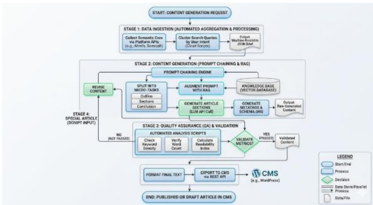
Рис. 1. Блок-схема конвеєра (Pipeline Process Flow)
