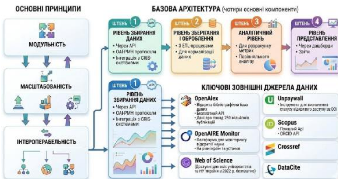
Рис. 2. Основні компоненти базової архітектури системи моніторингу
