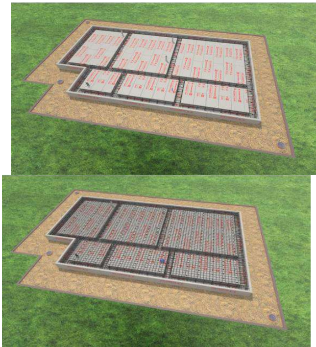
Рис. 5, 6 Армування ребер жорсткості
