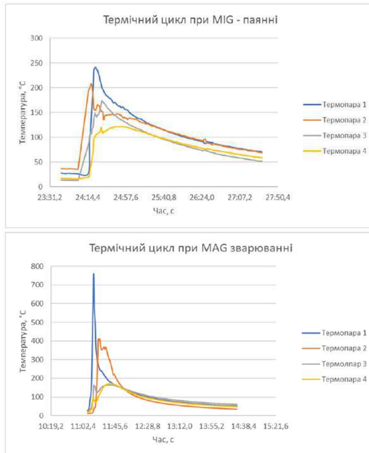
Рис. 1 Зміна температури при дуговому паянні та зварюванні
