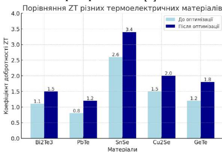
Рис. 2 Порівняння коефіцієнта добротності ( ZT ) різних термоелектричних матеріалів до та після оптимізації за допомогою штучного інтелекту
