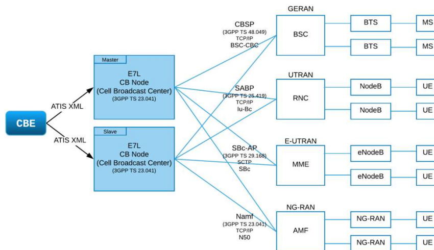
Рис. 1 Архітектура Cell Broadcast
