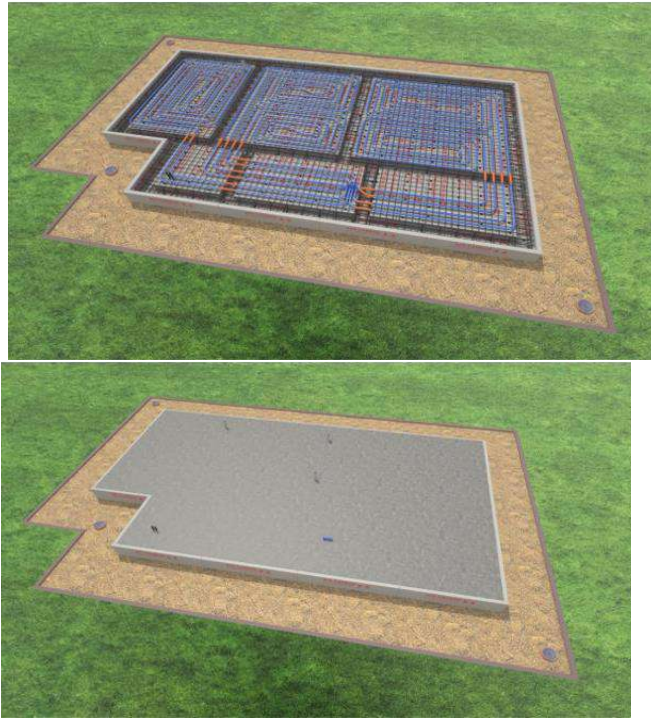
Рис. 7 Монтування труб підігріву підлоги
