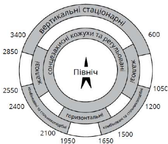
Рис. 1. Діаграма типів сонцезахисних пристроїв залежно від орієнтації фасадів
