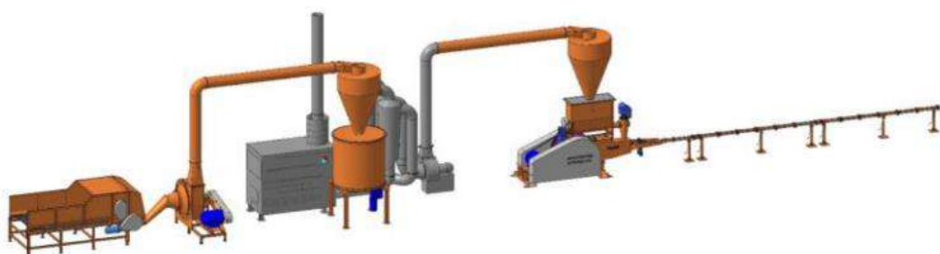
Рис. 5. Лінія брикетування від ПП «Брикетуючі технології»
