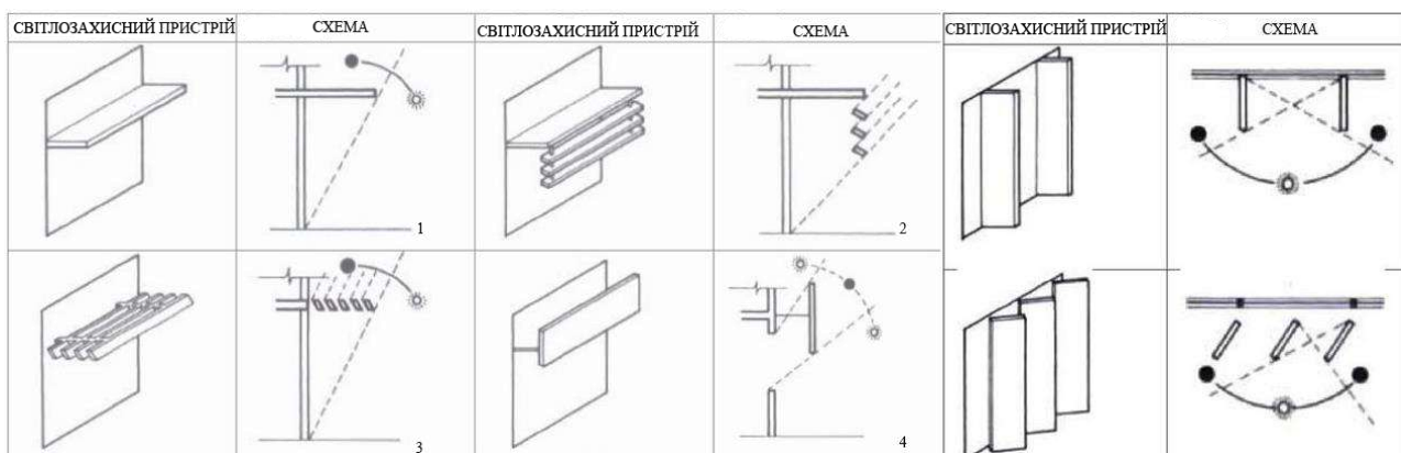
Рис. 2. Приклади сонцезахисних пристроїв [3]
