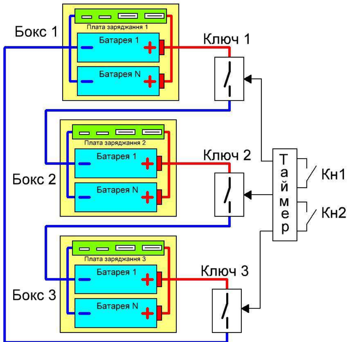
Рис. 2. Схема системи знешкодження
